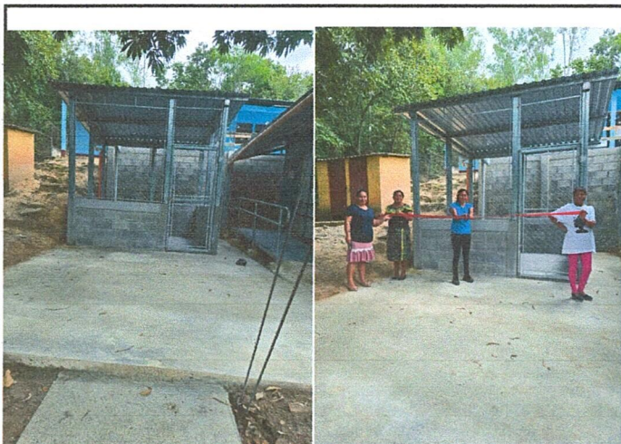
Foto 2: Suministro e instalación de cocina tipo pórtico, con puerta, polleton, plancha de 3 hornillas y chimenea
