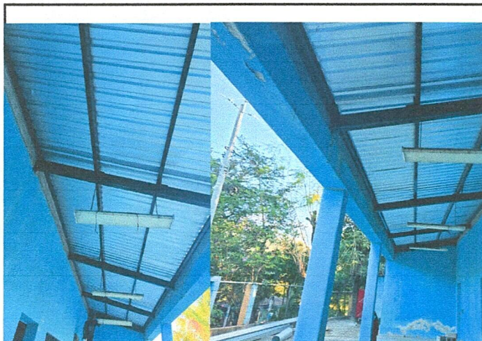
Foto 1: Cambio de lámina troquelada calibre 26, con lijado y pintado de la estructura metálica de techo existente, e instalación de canal metálico con bajadas pluviales en tubo PVC de 3" color blanco
